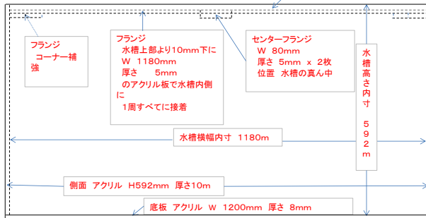
正面図面
