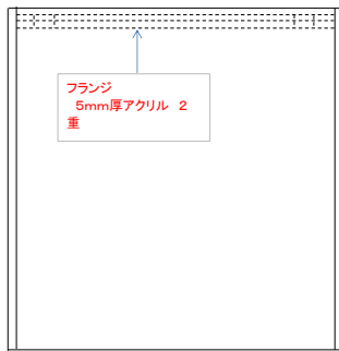
右側面図
