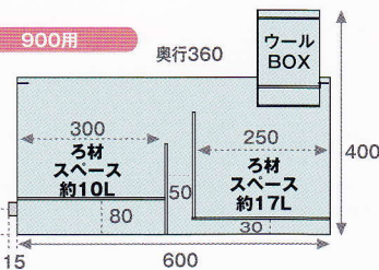
※設置例 リーフオクトパス IS-250
